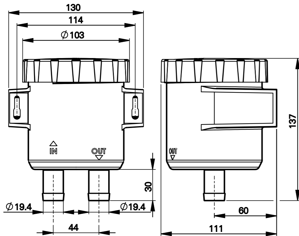
Hoofdafmetingen AG.010.20019
